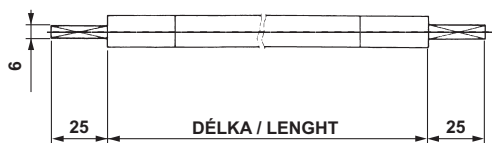
SPOJOVACÍ TYČ / CONNECTION ROD
